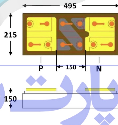
芯片外观尺寸图
