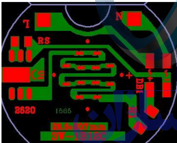
基板外观尺寸图
