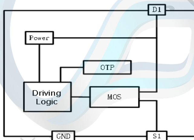
P3 RM9003AS Block Diagram
