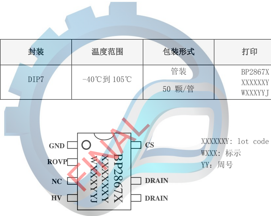
图 2 管脚封装图
